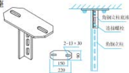
XQJ-H-02D角钢立柱底座 Angle-Steel Post Base
