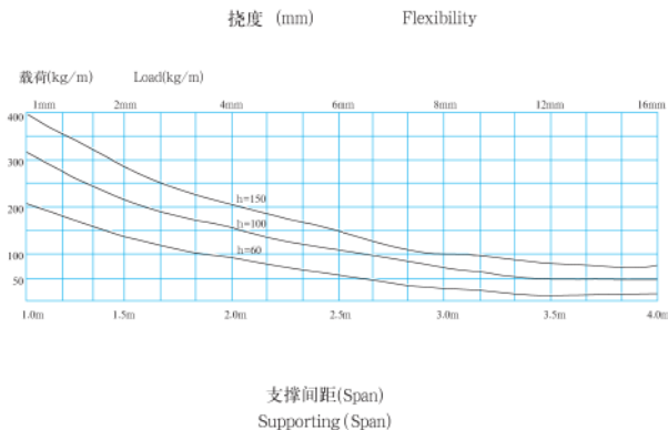
托盘式电缆桥架在不同跨距下最大允许均布载荷曲线图
