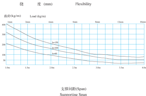
梯级式电缆桥架在不同跨距下最大允许均布载荷曲线图
