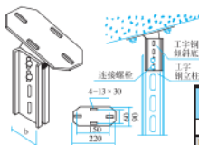
XQJ-H-03A工字钢倾斜底座 I-Steel Tilt
