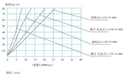
槽式、托盤式、梯級式載荷曲線 (B型)
