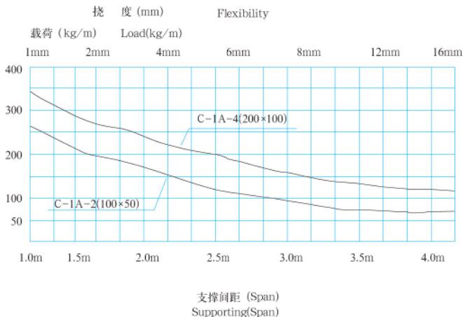
槽式电缆桥架在不同跨距下最大允许均布载荷曲线图
