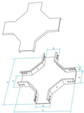
水平等径四通 XQJ-C-4A Horizontal Equant Cross Cable Tray
