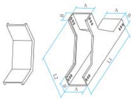
下垂直等径三通 XQJ-C-3C Lower Vertical Equant T-joint Cable Tray
