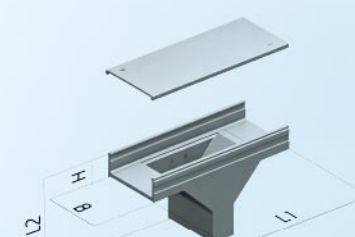
QJGHFF-C-03B型槽式上垂直三通
