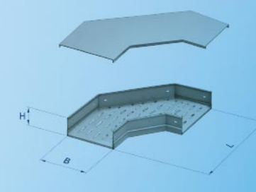
QJGHFF-P-02A型托盘式水平弯通
