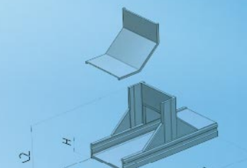
QJGHFF-C-03C型槽式下垂直三通
