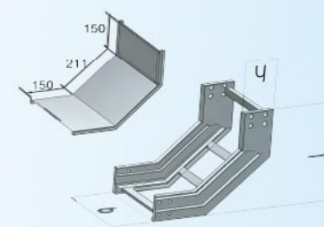
QJGHFF-T-05B型梯级式垂直下弯通
