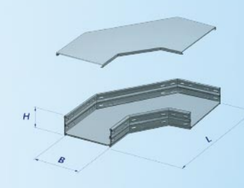
QJGHFF-C-02A型槽式水平弯通
