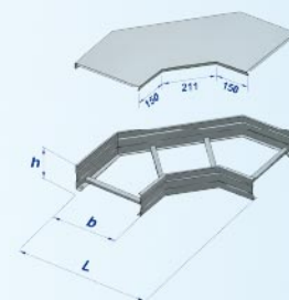
QJGHFF-T-02A型梯级式水平弯通
