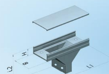
QJGHFF-P-03B型托盘式上垂直三通
