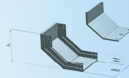
QJGHFF-C-05B型槽式垂直下弯通
